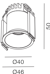
DL6019 IP44
