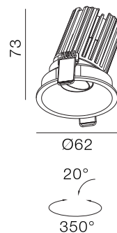
DL6010 IP54
